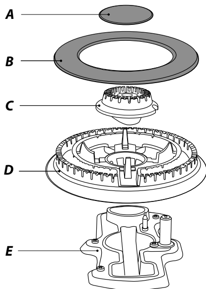
A – Inre brännarlock, B – Yttre brännarlock, C – Inre brännarkrona, D – Yttre brännarkrona, E – Wokbrännarens bas
