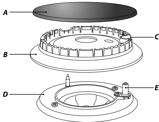
A – Lock, B – Krona, C – Skåra, D – Kropp, E – Elektrod
