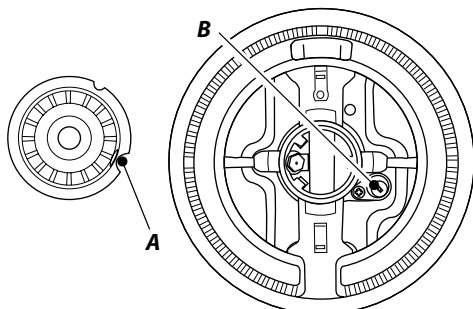
A – Elektrodskåra, B – Tändningselektrod
